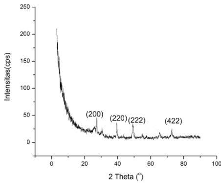
Gambar 4. Difraktogram lapisan tipis Sn(S 0,5 Te 0,5 ) sampel 3 dengan suhu substrat 500°C
