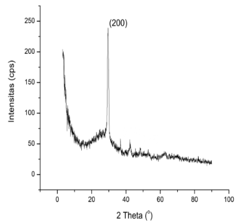
Gambar 2. Difraktogram lapisan tipis \text{Sn}(\text{S}_{0,5}\text{Te}_{0,5}) sampel 1 dengan suhu substrat 250^\circ\text{C}
