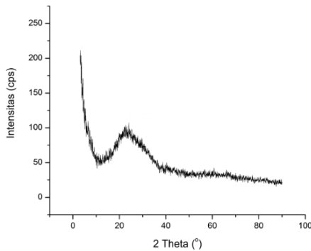
Gambar 5. Difraktogram lapisan tipis Sn(S 0,5 Te 0,5 ) sampel 4 dengan suhu substrat 600°C
