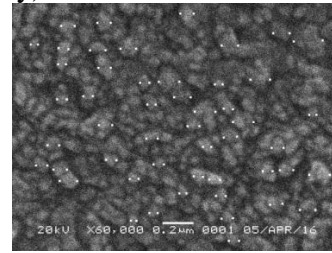
Gambar 7. Foto morfologi permukaan lapisan tipis Sn(S 0,5 Te 0,5 ) Sampel 3 hasil karakterisasi SEM dengan Perbesaran 60.000 kali yang sudah ditentukan ukurannya dengan diberi tanda pada program Paint
