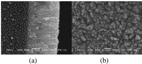
Gambar 6. Foto morfologi permukaan lapisan tipis Sn(S 0,5 Te 0,5 ) Sampel 3 hasil karakterisasi SEM dengan perbesaran (a) 30.000 kali dan (b) 60.000 kali
