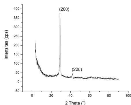
Gambar 3. Difraktogram lapisan tipis \text{Sn}(\text{S}_{0,5}\text{Te}_{0,5}) sampel 2 dengan suhu substrat 350^\circ\text{C}
