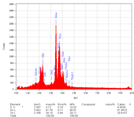
Gambar 9. Grafik antara intensitas dengan energi hasil karakterisasi EDS lapisan tipis Sn(S 0,5 Te 0,5 ) dengan teknik evaporasi vakum.
