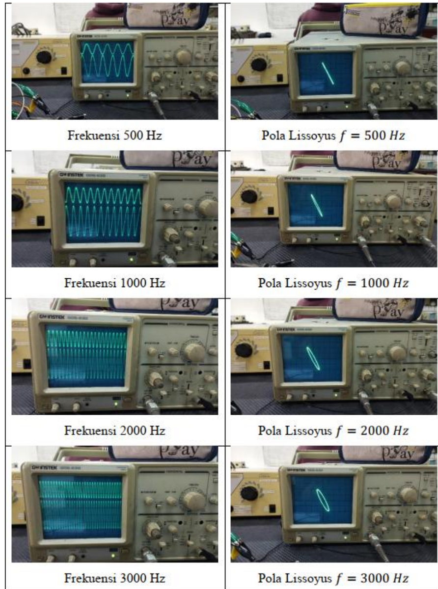
Gambar 4. Foto sinyal masukan dan sinyal keluaran serta pola Lissajous yang diukur dari rangkaian filter lolos rendah dengan konfigurasi R_1 = 1 \text{ k}\Omega , R_2 = 2,2 \text{ k}\Omega , dan C_2 = 10 \text{ nF} pada frekuensi 500–3000 Hz
