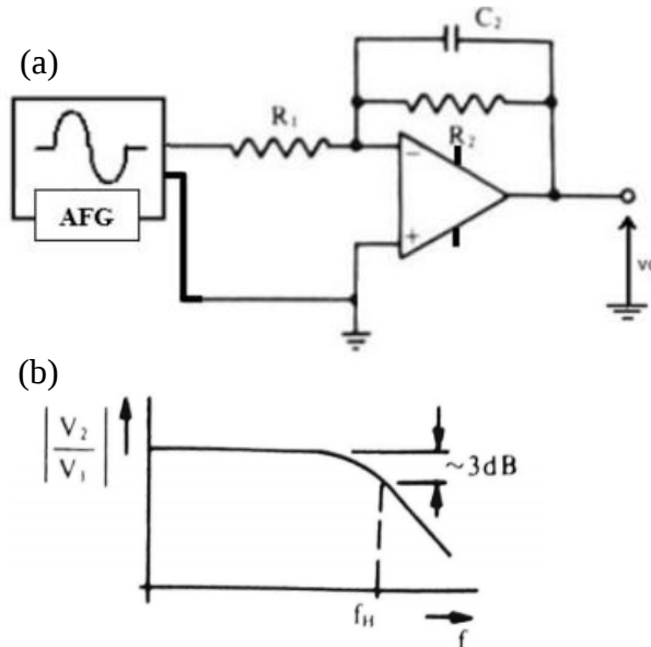
Gambar 2. (a) Diagram rangkaian dan (b) karakteristik frekuensi filter lolos rendah:
