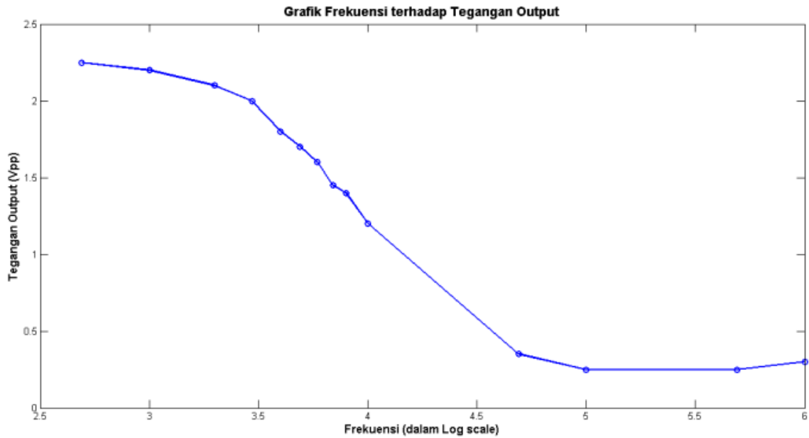
Gambar 5. Grafik respons frekuensi filter lolos rendah yang menunjukkan hubungan antara tegangan output (Vpp) dengan frekuensi (dalam skala logaritmik)
