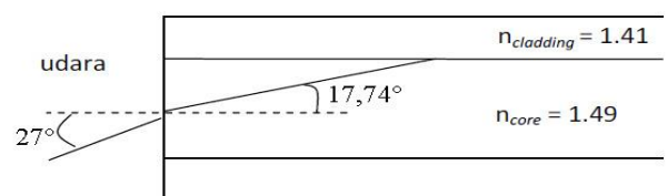
Gambar9. Sudut datang dalam bidang batas core dan cladding
