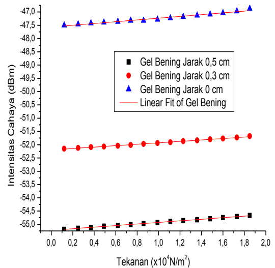
Gambar 4. Grafik Hubungan Antara Intensitas Cahaya Terhadap Tekanan Dengan Gel Pulpen Bening
