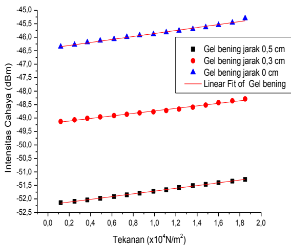
Gambar 7. Grafik Hubungan Antara Intensitas Cahaya Terhadap Tekanan Dengan Gel Rambut Kuning
