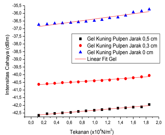
Gambar 5. Grafik Hubungan Antara Intensitas Cahaya Terhadap Tekanan Dengan Gel Pulpen Kuning
