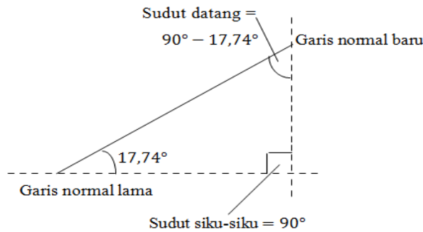
Gambar 10. Sudut datang dalam bidang batas core dan cladding
