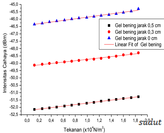
Gambar 6. Grafik Hubungan Antara Intensitas Cahaya Terhadap Tekanan Dengan Gel Rambut Bening
