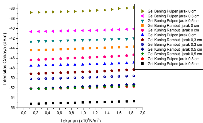
Gambar 3. Grafik Hubungan Antara Tekanan dan Intensitas Cahaya Pada Gel Rambut Dan Gel Pulpen
