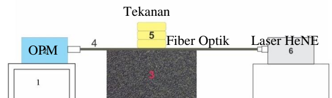
Gambar 2. Desain alat penelitian
