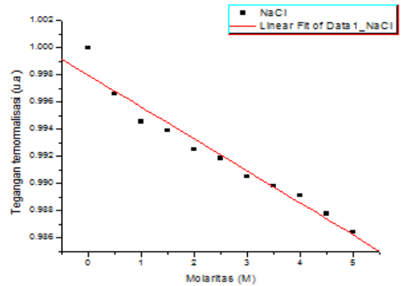
Gambar 5. Grafik hubungan antara konsentrasi larutan (M) terhadap tegangan keluaran ternormalisasi (u.a) pada larutan Garam (NaCl)
