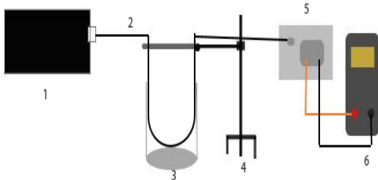
Gambar 2. Desain alat penelitian.
