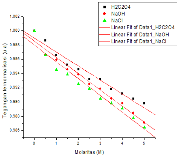
Gambar 6. Grafik Hubungan antara tegangan keluaran ternormalisasi (u.a) terhadap konsentrasi larutan asam oksalat (H 2 C 2 O 4 ), larutan natrium hidroksida (NaOH) dan larutan garam (NaCl).
