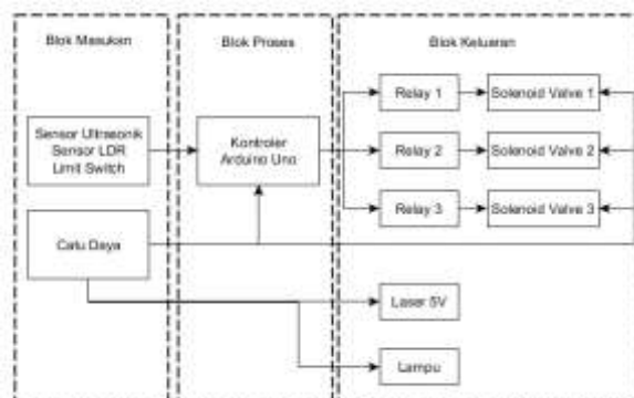
Gambar 1. Blok Diagram Rangkaian Alat
