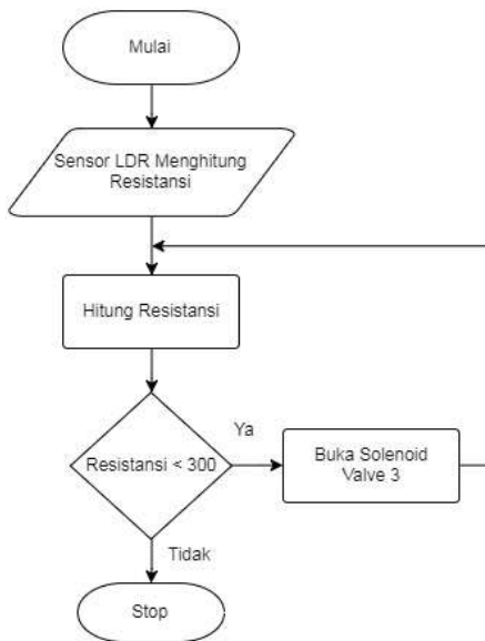
Gambar 7. Flowchart Limit Switch Pada Lampu
