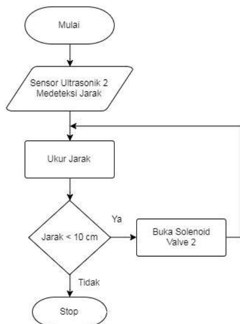
Gambar 5. Flowchart Program Sensor Ultrasonik Pada Shower
