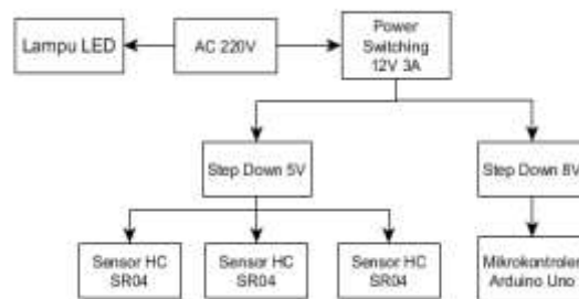
Gambar 2. Rangkaian Catu Daya dan sensor
