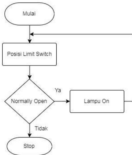
Gambar 6. Flowchart Program Sensor LDR Pada Closet
