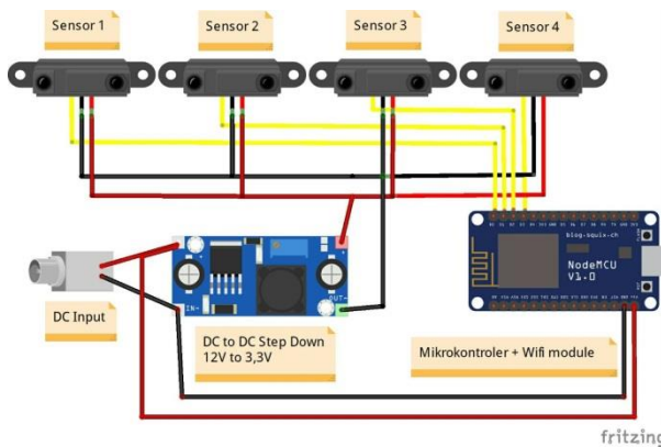
Gambar 2. Rangkaian Alat
