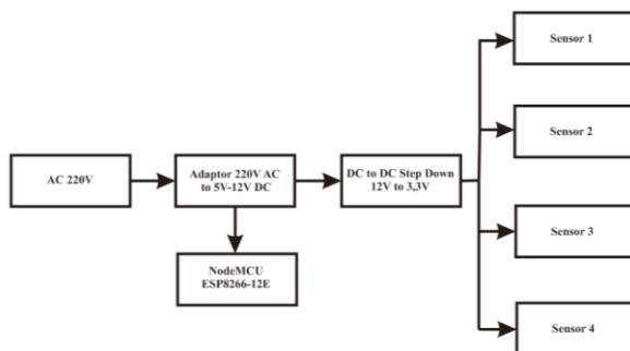
Gambar 3. Blok Diagram Catu Daya
