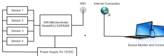
Gambar 1. Diagram Blok Rangkaian
