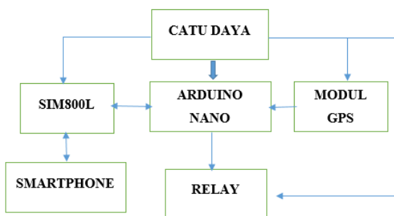
Gambar 2. Blok Diagram Utama Sistem
