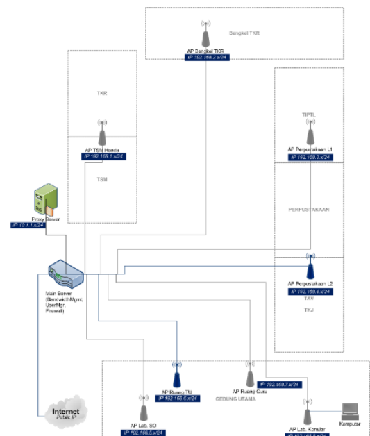
Gambar Usulan Perbaikan Jaringan
