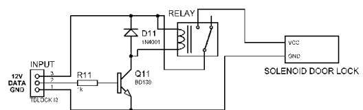
Gambar 4. Rangkaian Relay dengan Solenoid door lock
