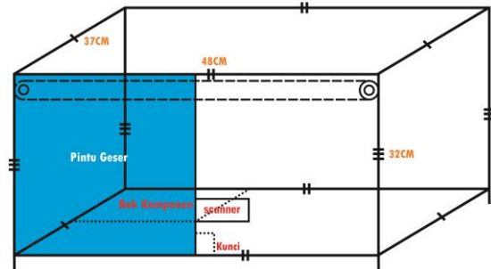
Gambar 7. Desain Box Alat
