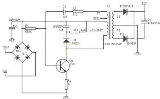
Gambar 2. Rangkaian Catu Daya
